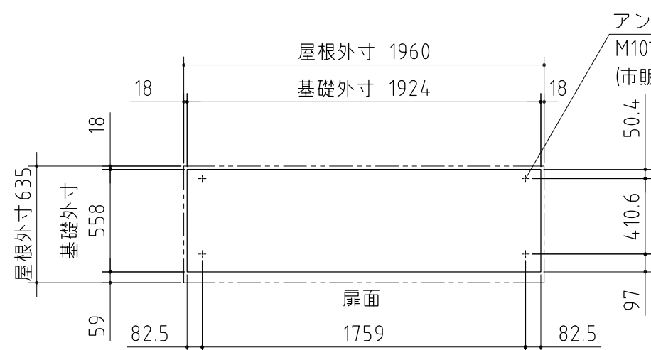
ベタ基礎図
